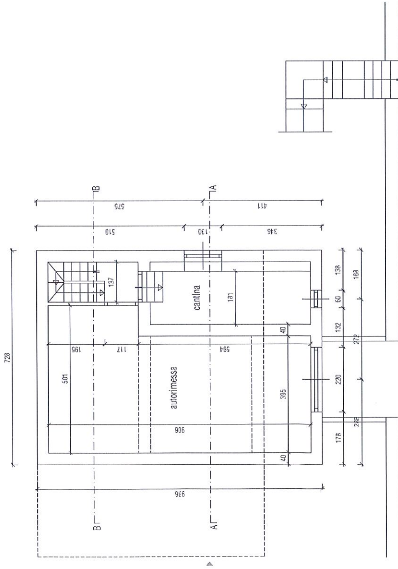
PIANTA PIANO INTERRATO
